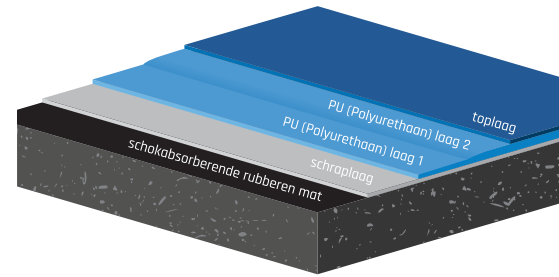
Sportvloer opbouw
